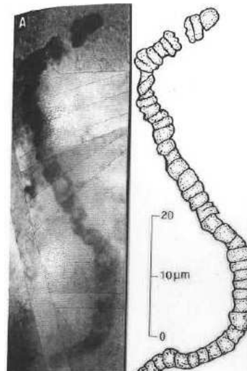
Photographie d'une structure retrouvée dans une lame mince de stromatolithe fossile (Pilbara, Australie)
